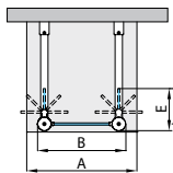
FUT2 + stabilizační vzpěry
