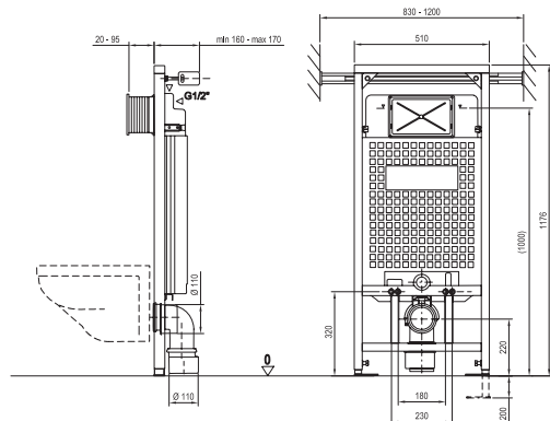
Předstěnový instalační modul G se vzpěrrou
