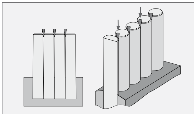
Použití distančnicku pro vyrovnání kónicity palisád
