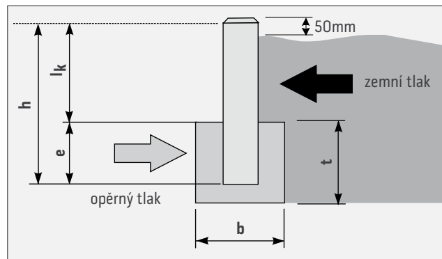
Technické údaje pro zabudování palisád
